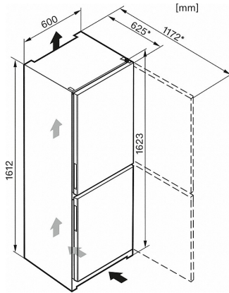
KD26022Sws, KD26022Sedt/cs, (schéma) (*note en bas de page)
